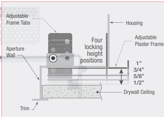
VF150 TRIM DETAIL
