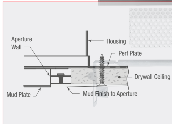
VF100 TRIMLESS DETAIL
